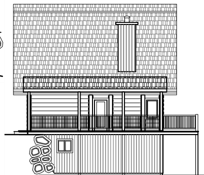
ÉLÉVATION GAUCHE
