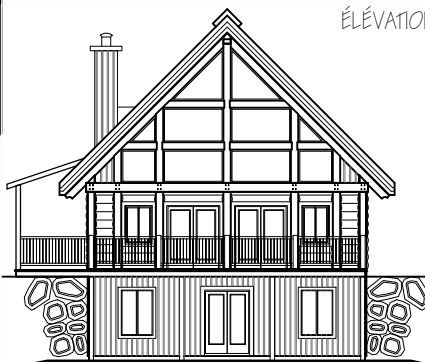
ÉLÉVATION AVANT
