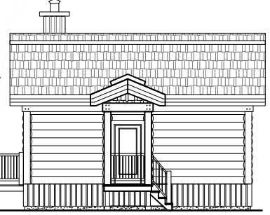
ÉLEVATION GAUCHE
