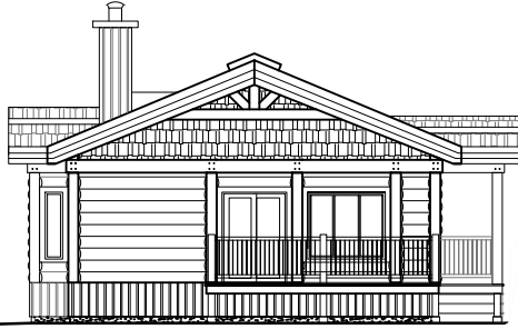
ÉLEVATION AVANT
